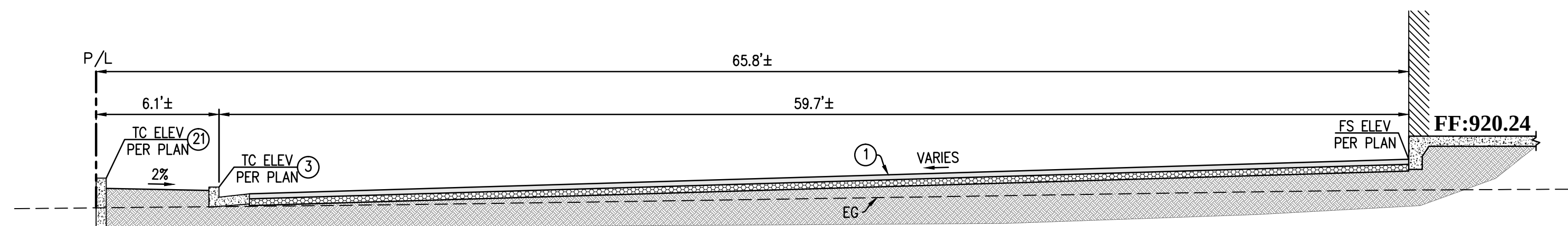
SECTION D-D SCALE: 1"=5'
