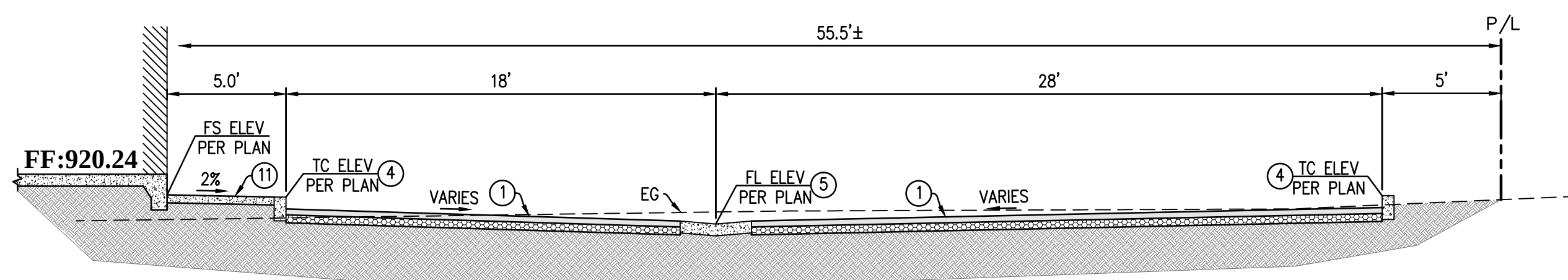
SECTION C-C SCALE: 1"=5'
