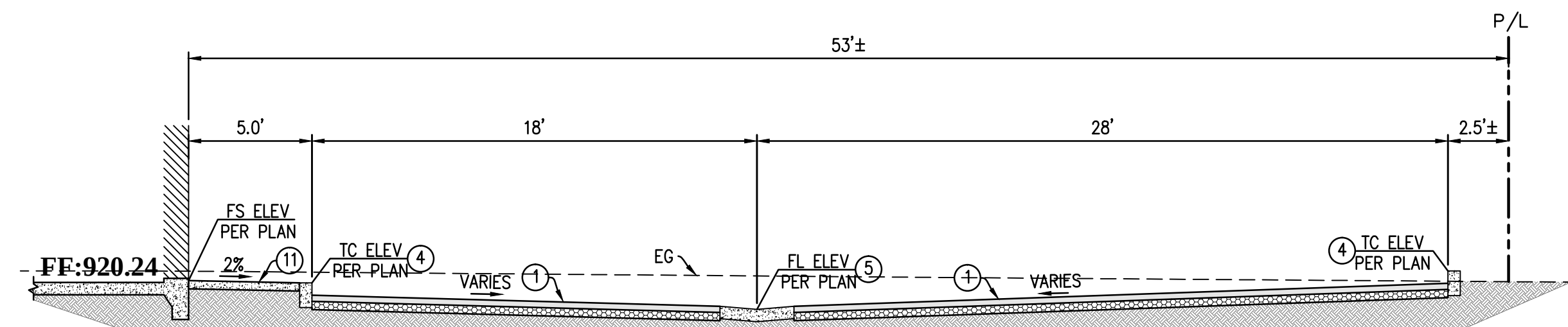
SECTION G-G SCALE: 1"=5'
