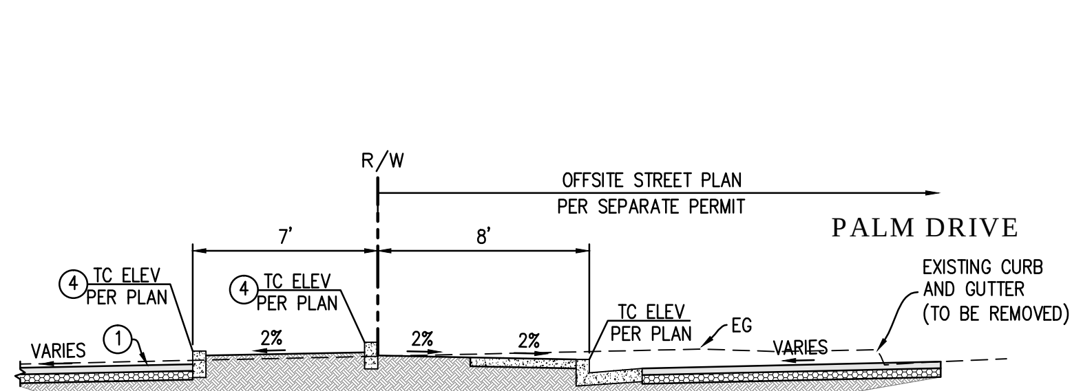
SECTION A-A SCALE: 1"=5'
