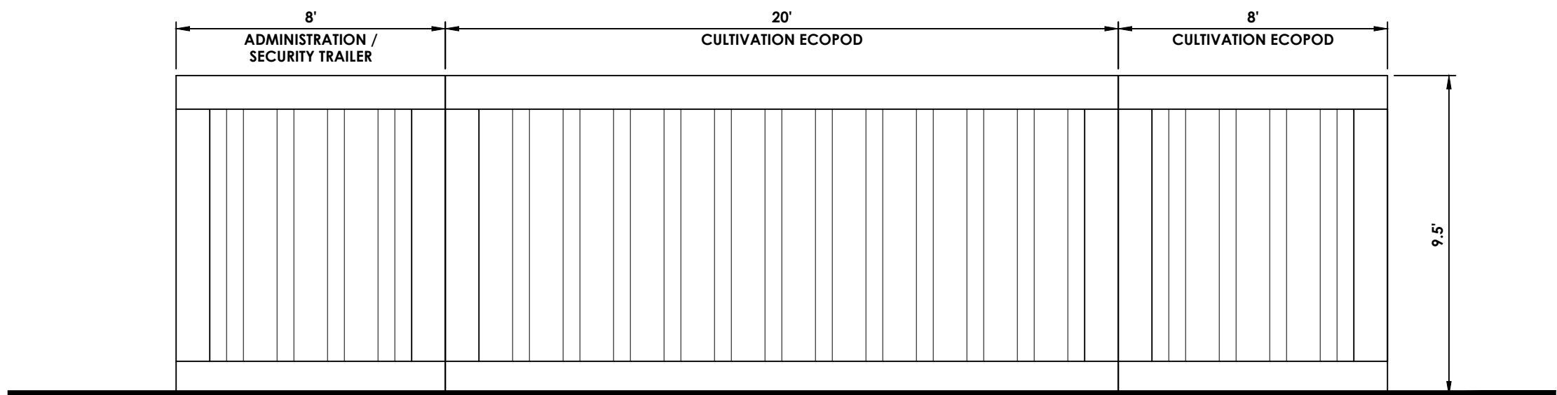
EAST ELEVATION N.T.S.
